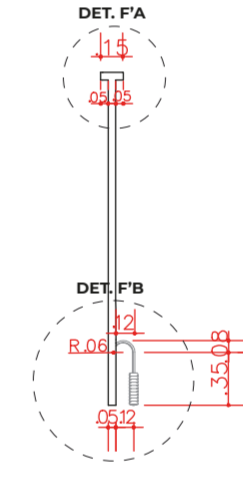
VISTA LAT. ESC.: 1:50
