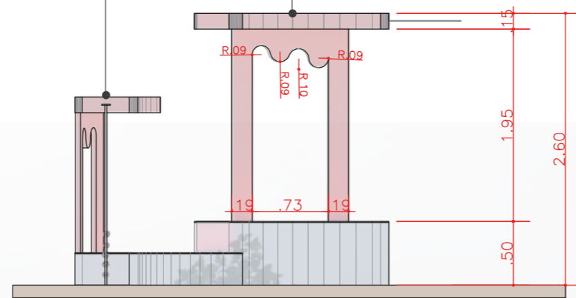
VISTA B ESC.: 1:50
