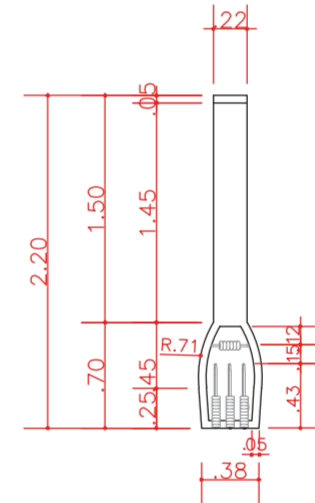
VISTA FRONTAL ESC.: 1:50
