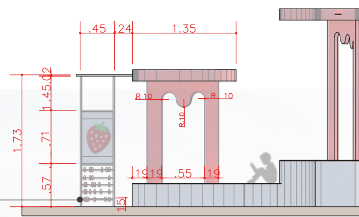
VISTA A ESC.: 1:50
