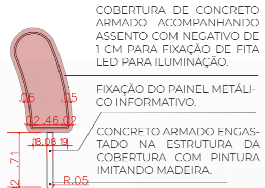
DET. C - COBERTURA ESC.: 1:50
