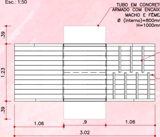
Vista Superior - "Sky Adventure" Esc.: 1:50
