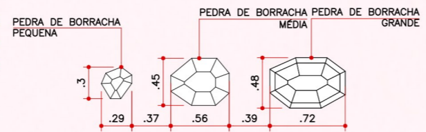
Vista Superior - "Pedras do Pulo" Esc.: 1:50
