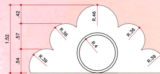
Vista Frontal - "Sky Adventure" Esc.: 1:50
