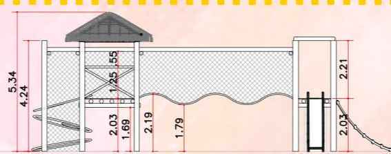
Vista Lateral - Bem Aventurado's ESC.: 1:200
