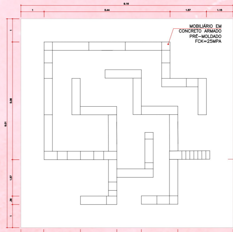
Vista Superior - "Labirinto Mágico" ESC.: 1:100
