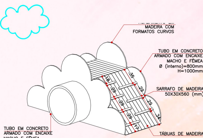
Perspectiva - "Sky Adventure" SEM ESCALA
