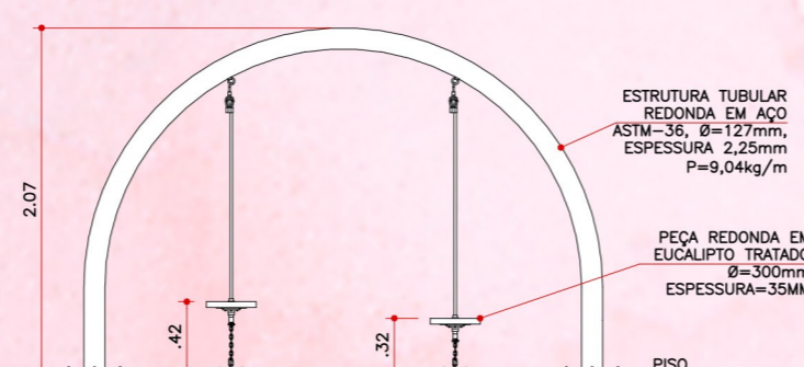
Vista Frontal - "Abraça corda" ESC.: 1:50
