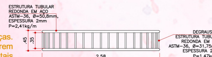
Vista Superior - Escada em Arco ESC.: 1:50
