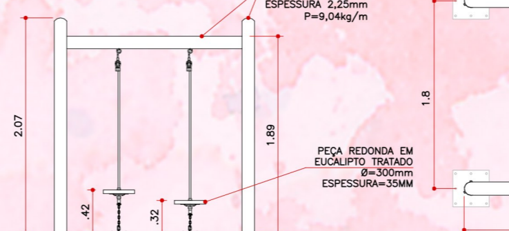
Vista Lateral - "Abraça corda" ESC.: 1:50
