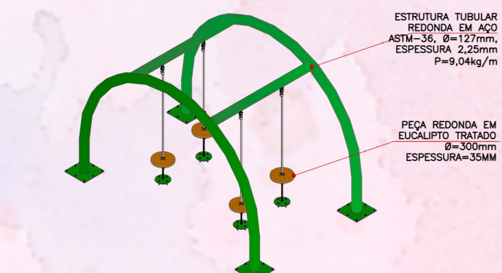
Perspectiva - "Abraça corda" SEM ESCALA
