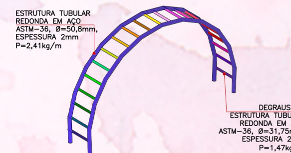
Perspectiva - Escada em Arco SEM ESCALA
