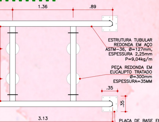
Vista Superior - "Abraça corda" ESC.: 1:50
