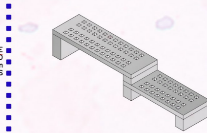
Perspectiva - Banco Furado ESTRUTURA EM CONCRETO PRÉ-MOLDADO ESC.: 1:50
