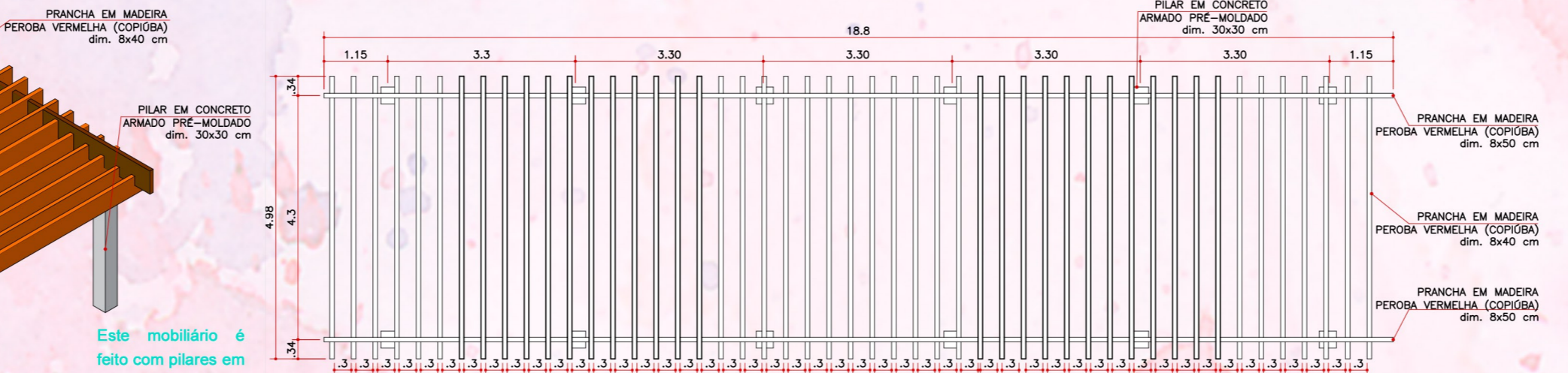
Vista Lateral - "Pergolado Dançante" OBS.: AS PRANHAS DE DIM. 8 X 40 cm SERÃO INSTALADA COM DIFERENÇA DE ALTURA DE 5CM ENTRE CADA UMA, CONFORME PROJETO. ESC.: 1:100
